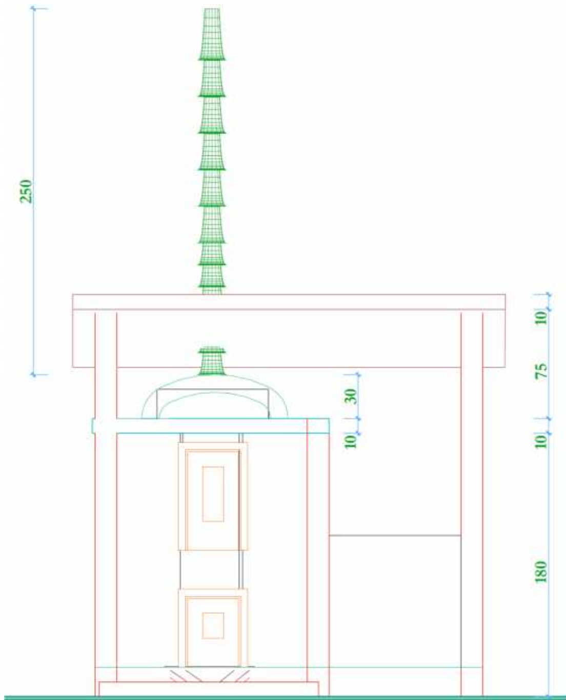
COUPE B-B
