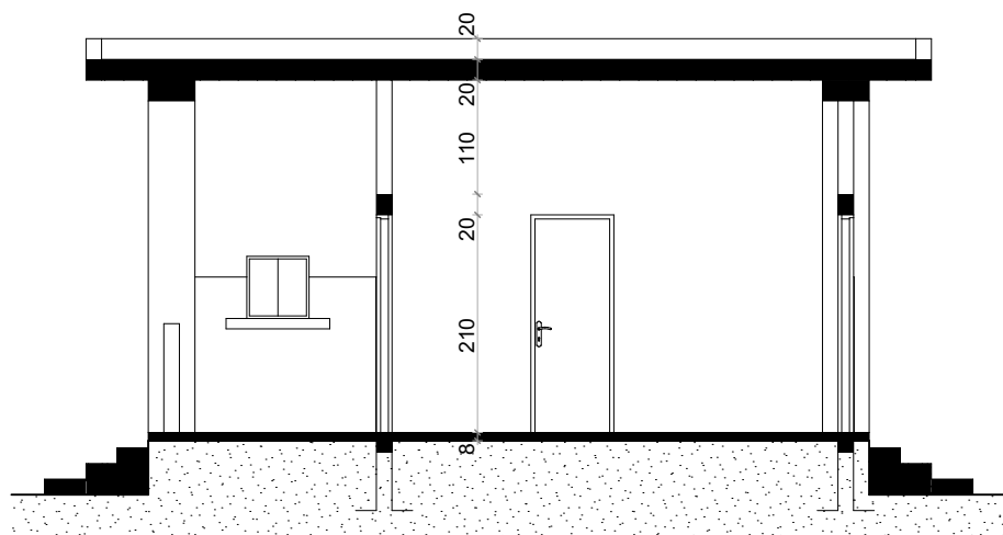
B - B
