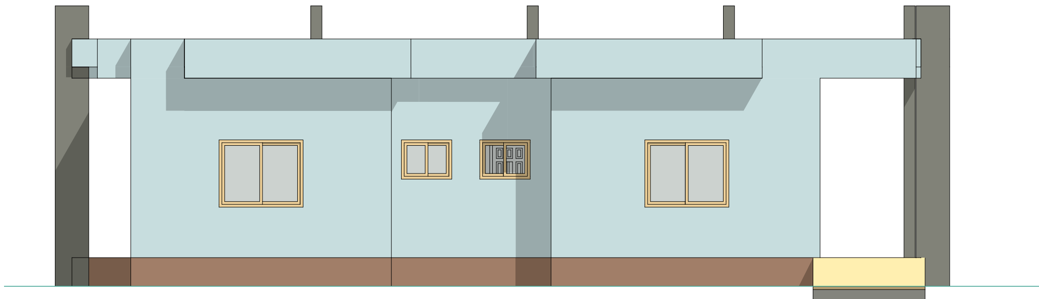
FACADE LATÉRALE GAUCHE MATERNITE TYPE CSA
