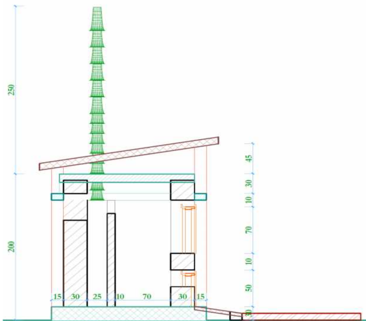
COUPE A-A
