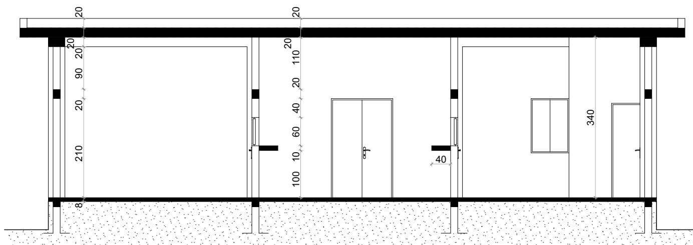
A - A
