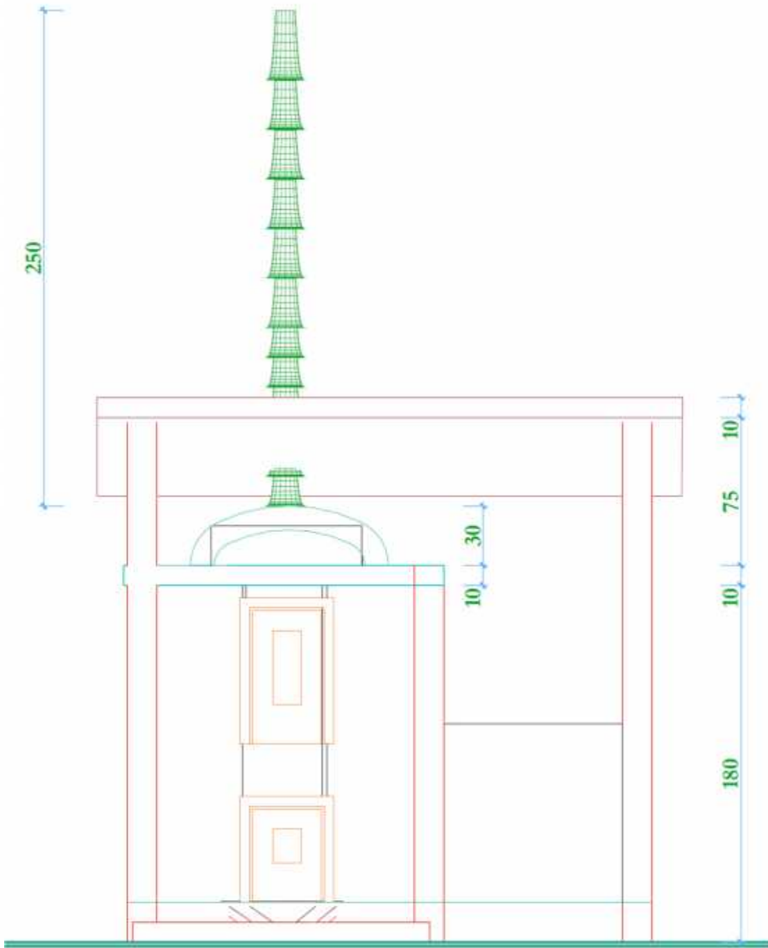
COUPE B-B
