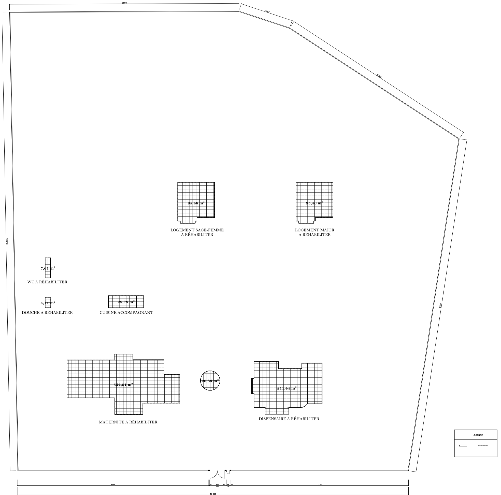
PLAN DE MASSE ETAT DES LIEUX CS ADJIDO
