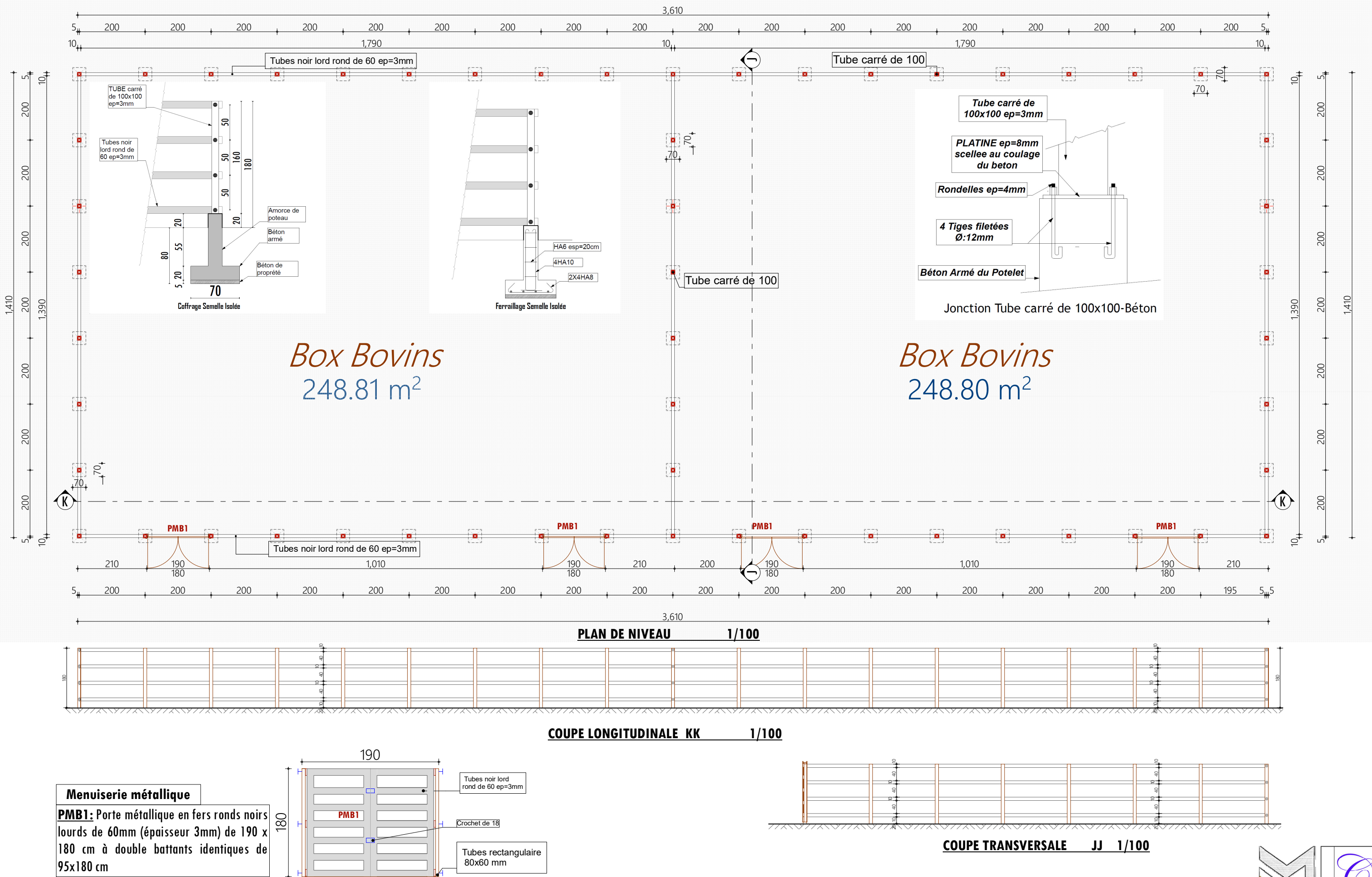
PLAN TYPE - MARCHE A BETAIL- BOX BOVINS
