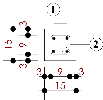
COUPE SUR POTEAU RAIDISSEUR R (15x15)
