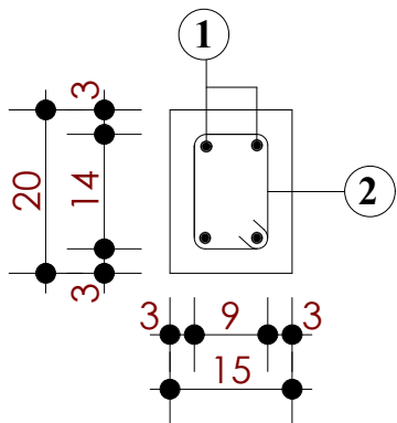
COUPE SUR CHAINAGE BAS CH (15x20)
