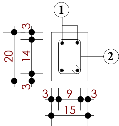
COUPE SUR CHAINAGE HAUT CH (15x20)
