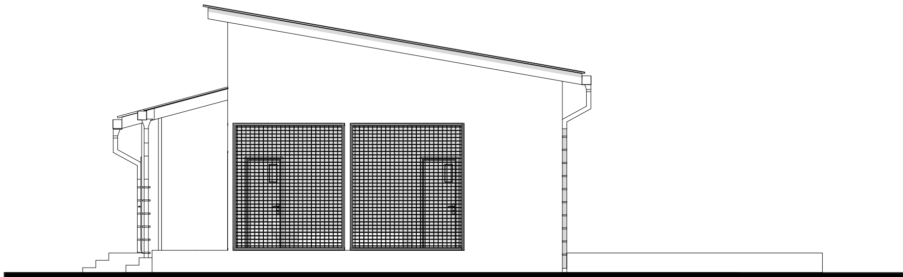
FACADE LATÉRALE GAUCHE
