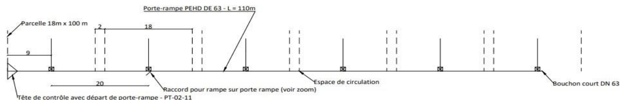
Porte rampe avec 6 raccords unilatéraux pour rampe (module 1x6) - Vue en plan
