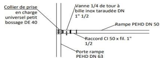
Zoom sur un raccord pour rampe - vue en plan
