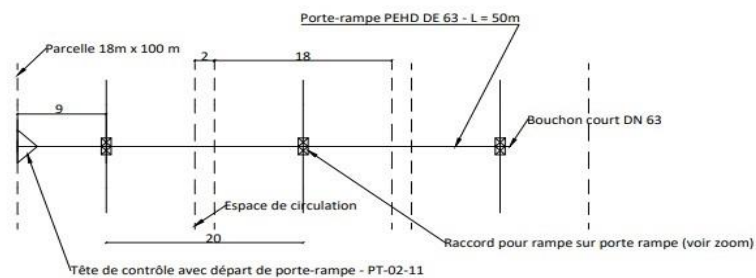
Porte rampe avec 6 raccords pour rampe (module 2x3) - Vue en plan
