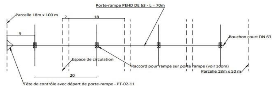
Porte rampe avec 8 raccords pour rampe (module 2x4) - Vue en plan
