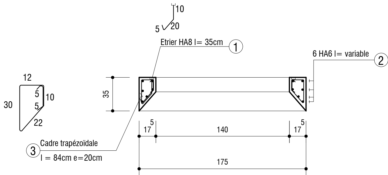
Coupe 1-1
