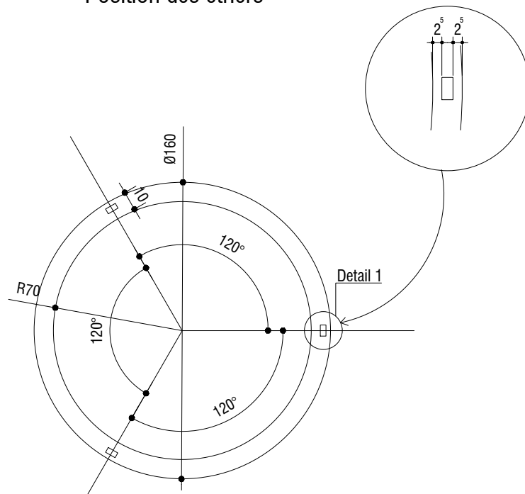
Position des étriers
