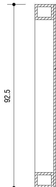
Coupe A - A
