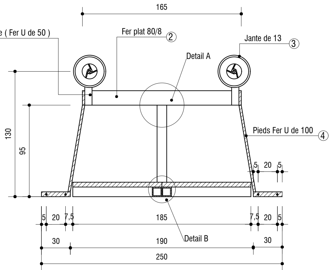
Coupe B-B
