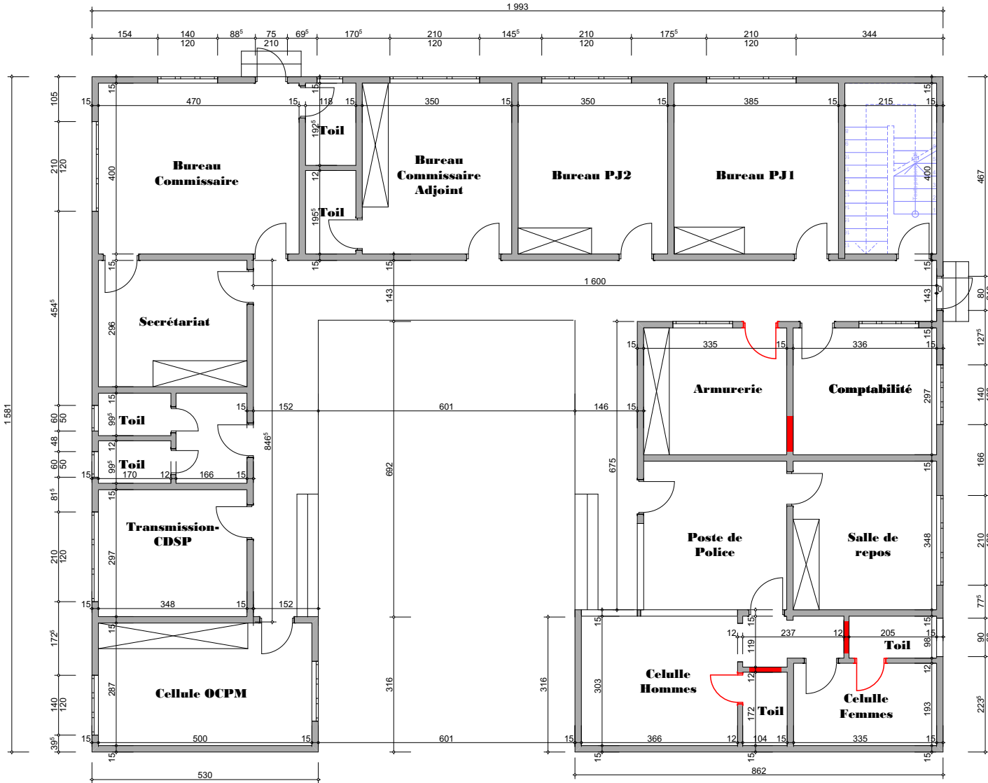
PLAN MODIFIE COMMISSARIAT DU 2EME ARRONDISSEMENT DE PARAKOU
