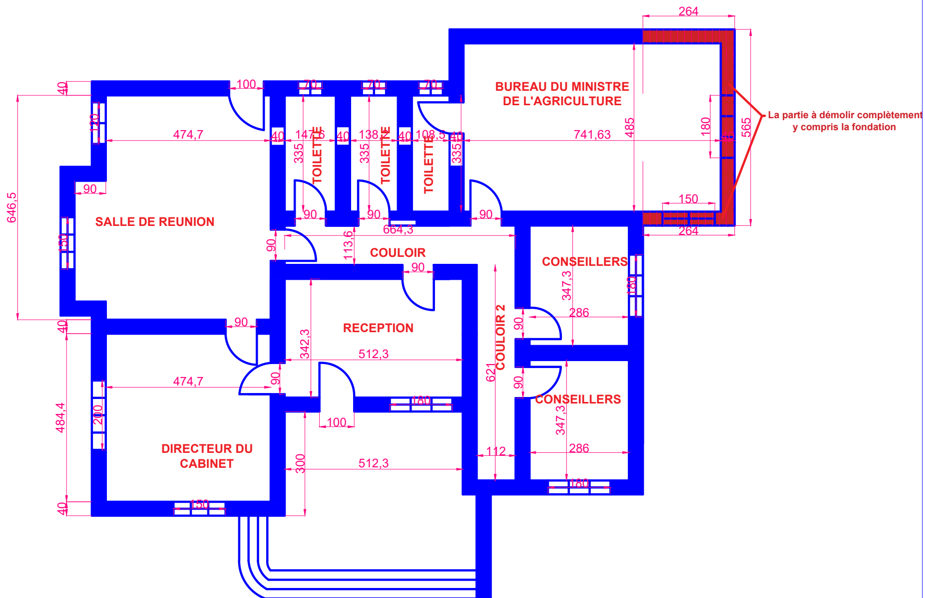
VUE EN PLAN BUREAU DU MINISTRE
