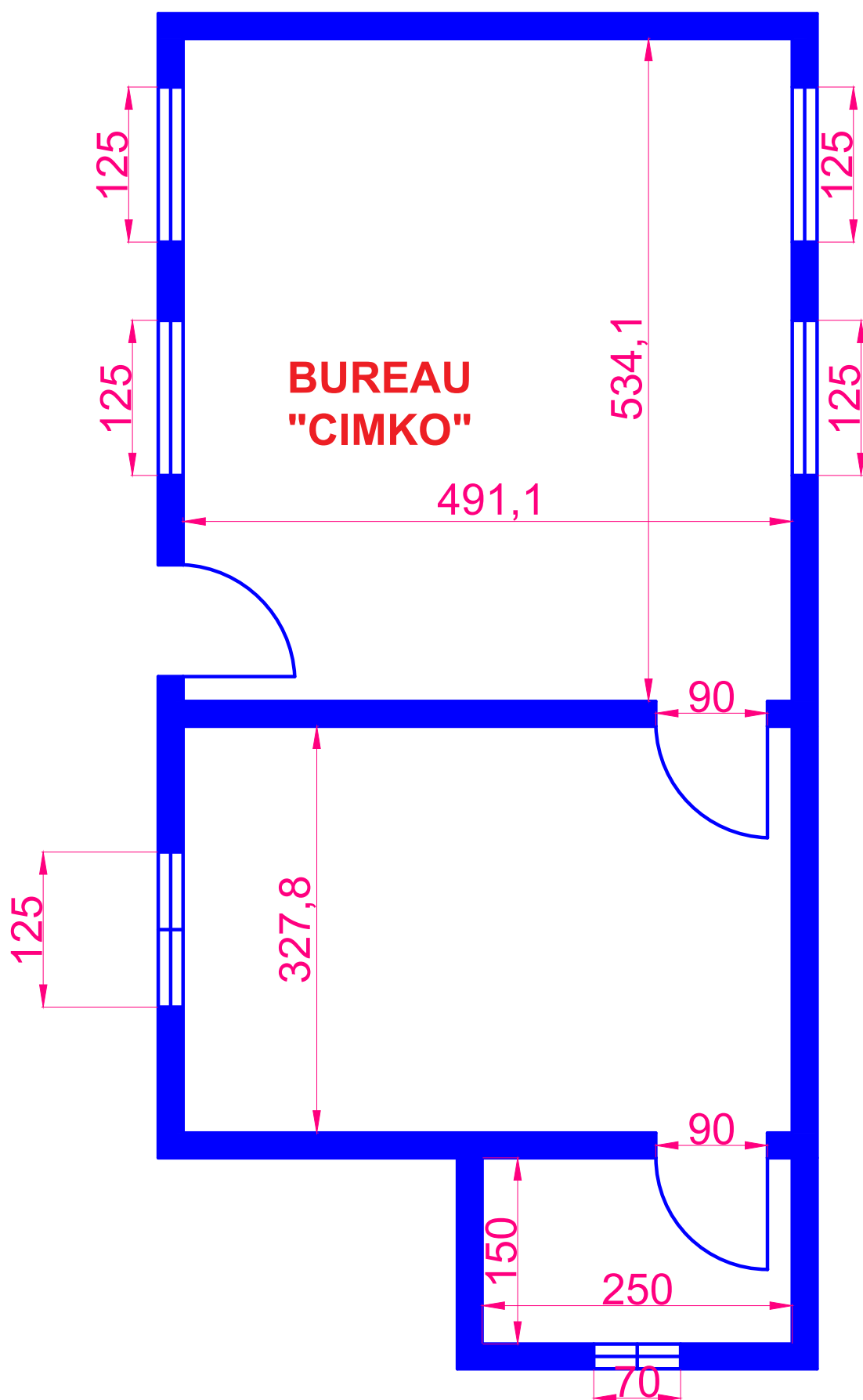
VUE EN PLAN BUREAU "CIMKO"
