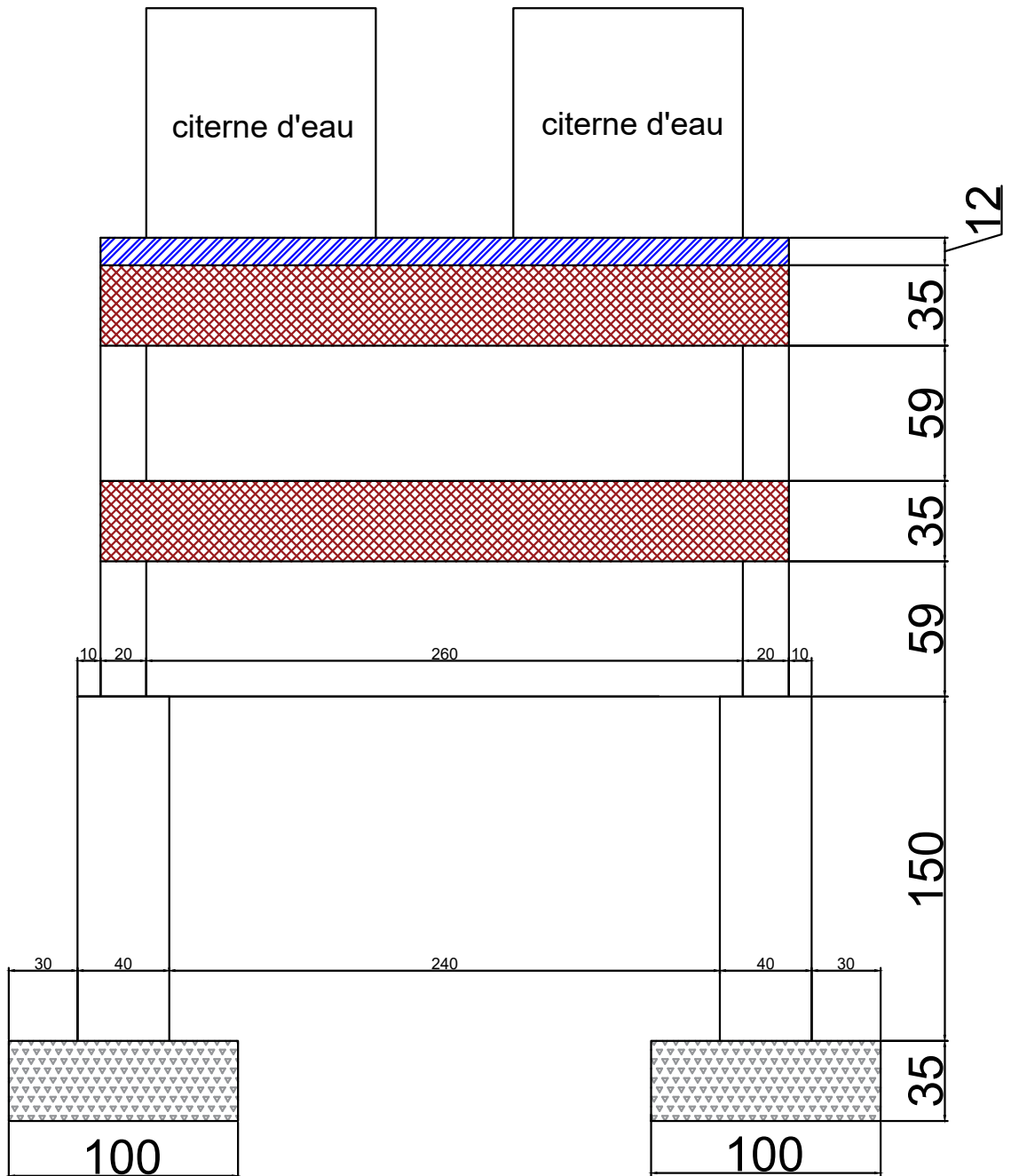
support citerne d'eau en B.A
