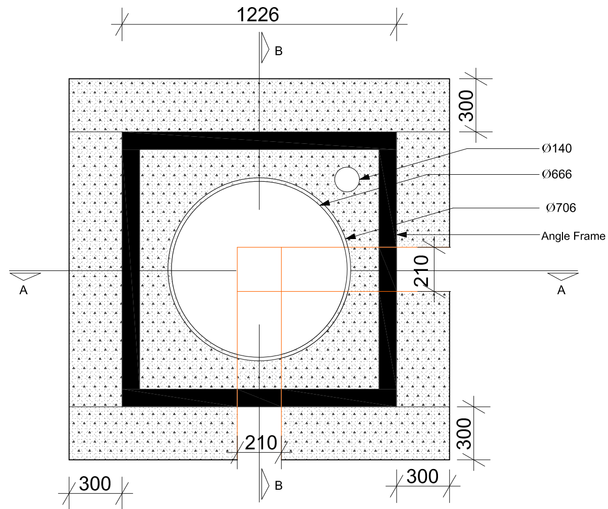
PLAN VIEW SCALE: 1:15
