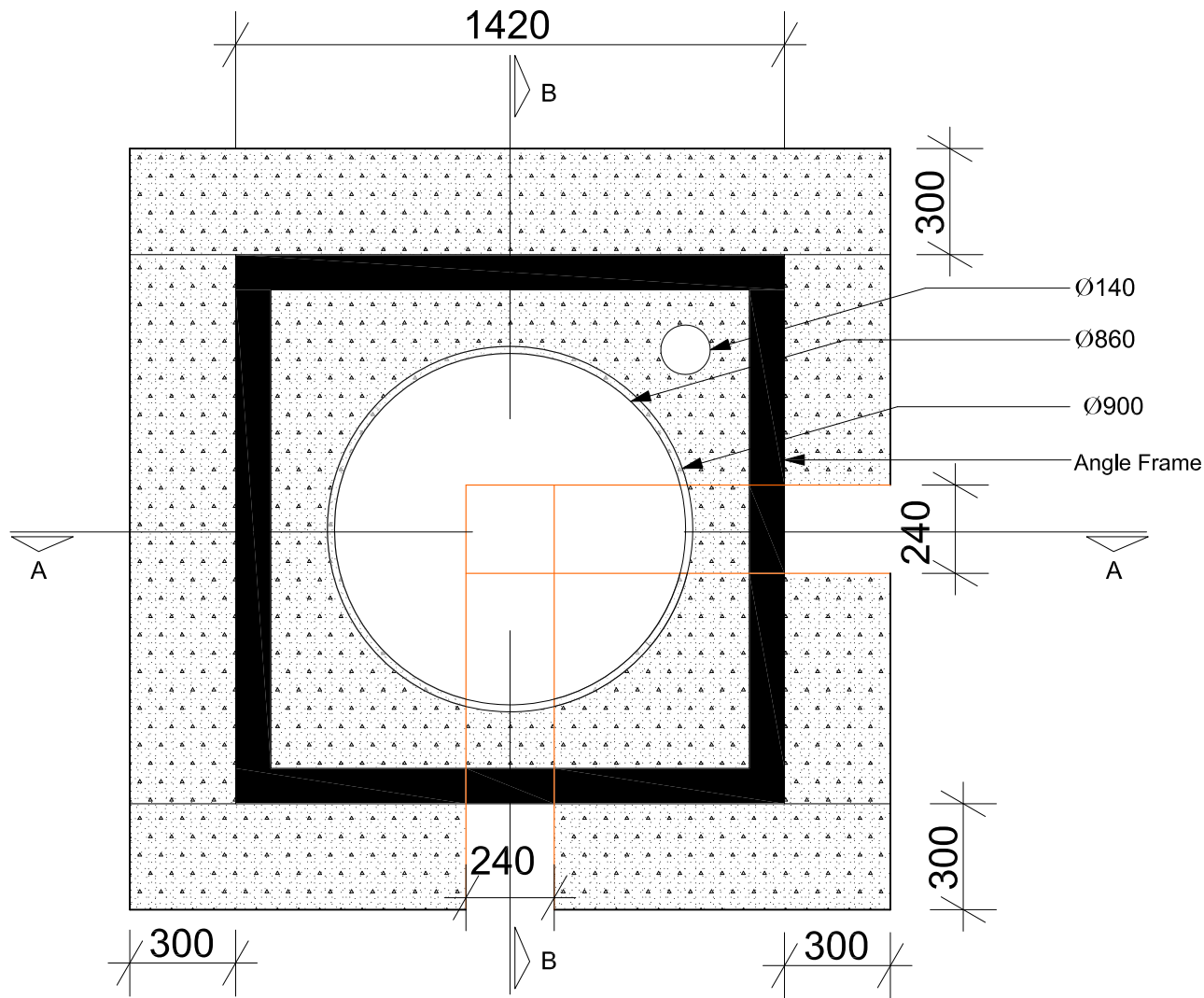
PLAN VIEW SCALE: 1:18
