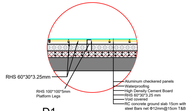
D1 Scale 1:50
