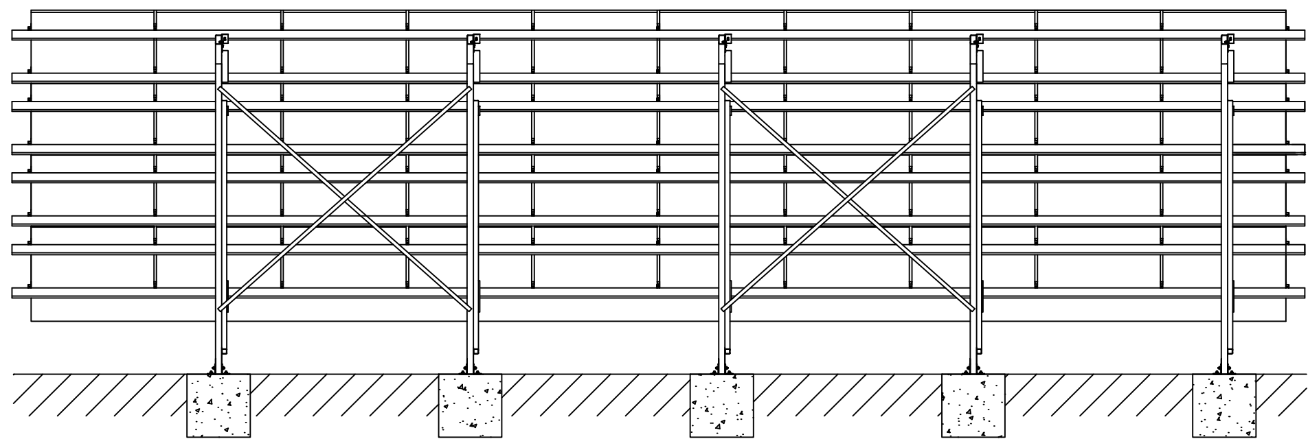
Vista traseira
