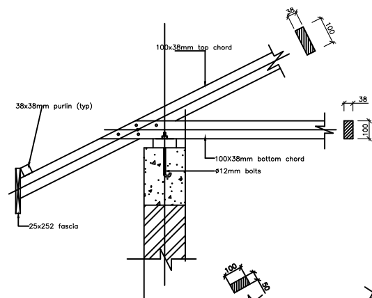
DETAIL D1
