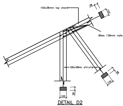
DETAIL D2
