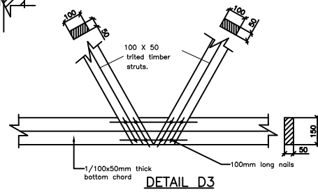
DETAIL D3
