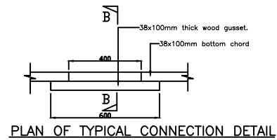
DETAIL D5
