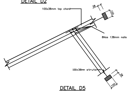
DETAIL D5
