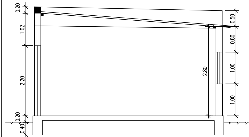
COUPE AA
