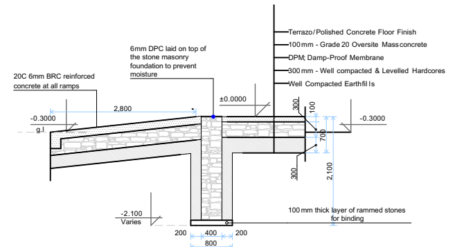
SECTION 2a
