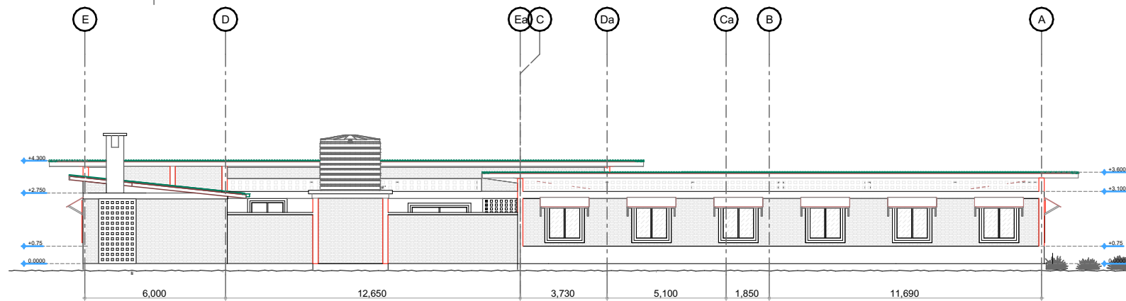
L.H.S ELEVATION
