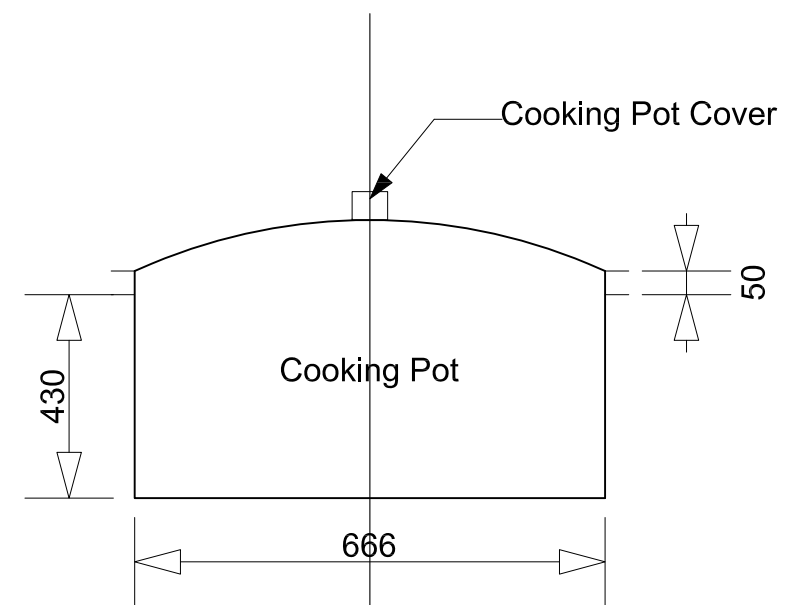
SCALE: 1: 10
