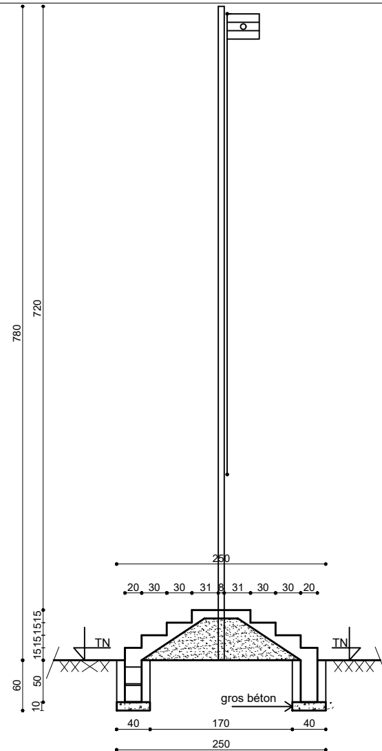
Coupe A-A
