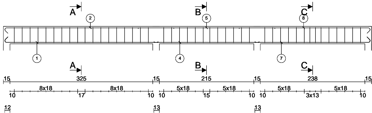
Élévation Echelle=1/44
