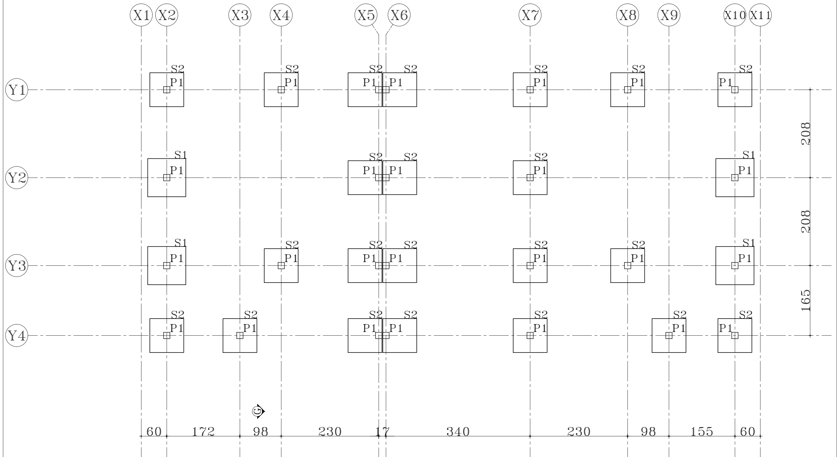
ENSEMBLE FONDATIONS SEMELLES COFFRAGE -1.00m/TN
