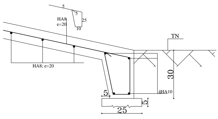
COUPE DETAIL Be2 FERRAILAGE
