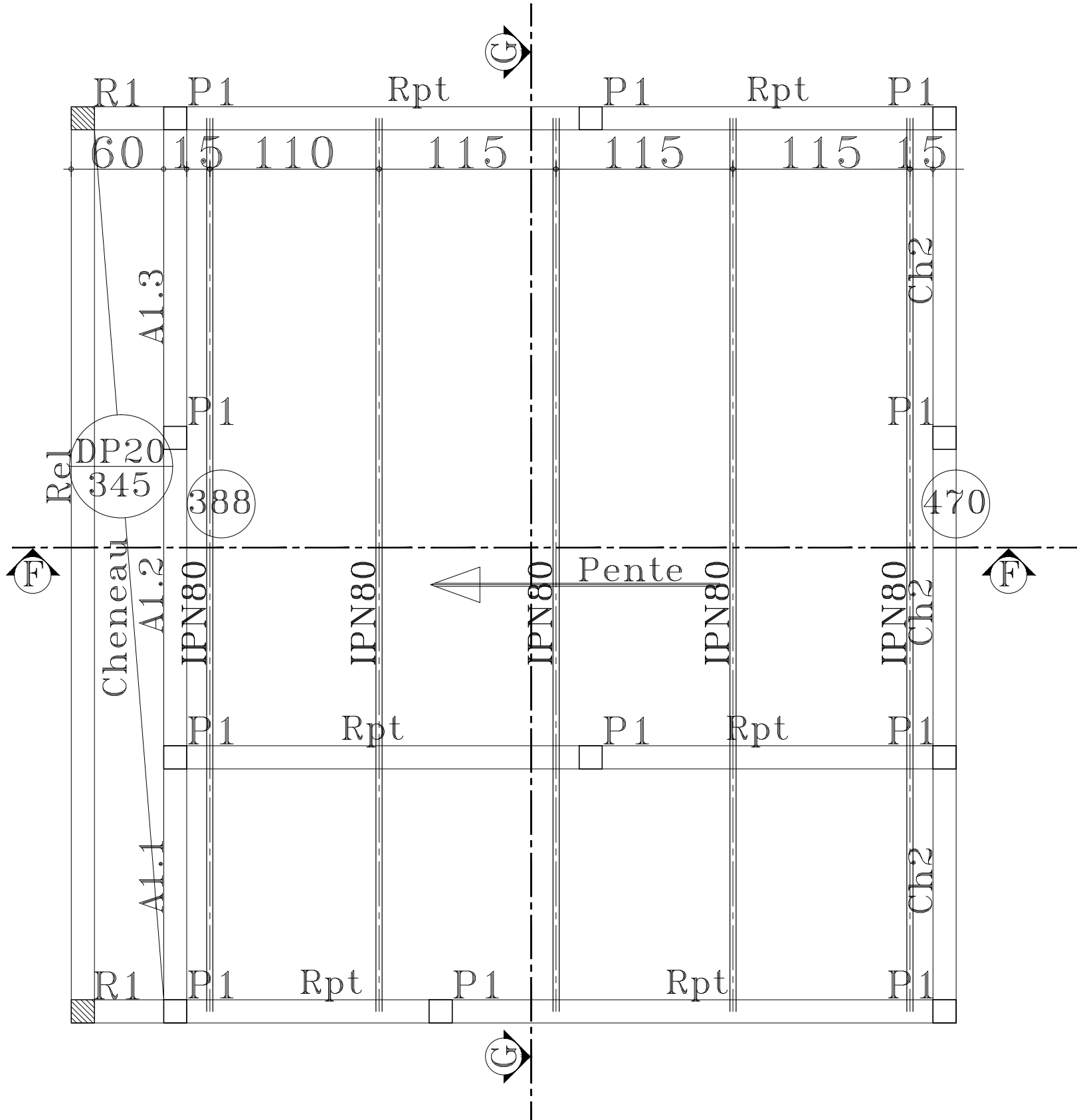
COFFRAGE TOITURE LEGERE VAR.m/TN
