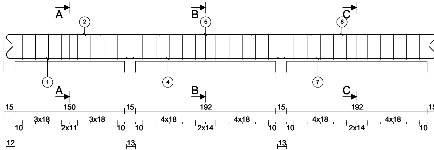
Elévation Echelle=1/32
