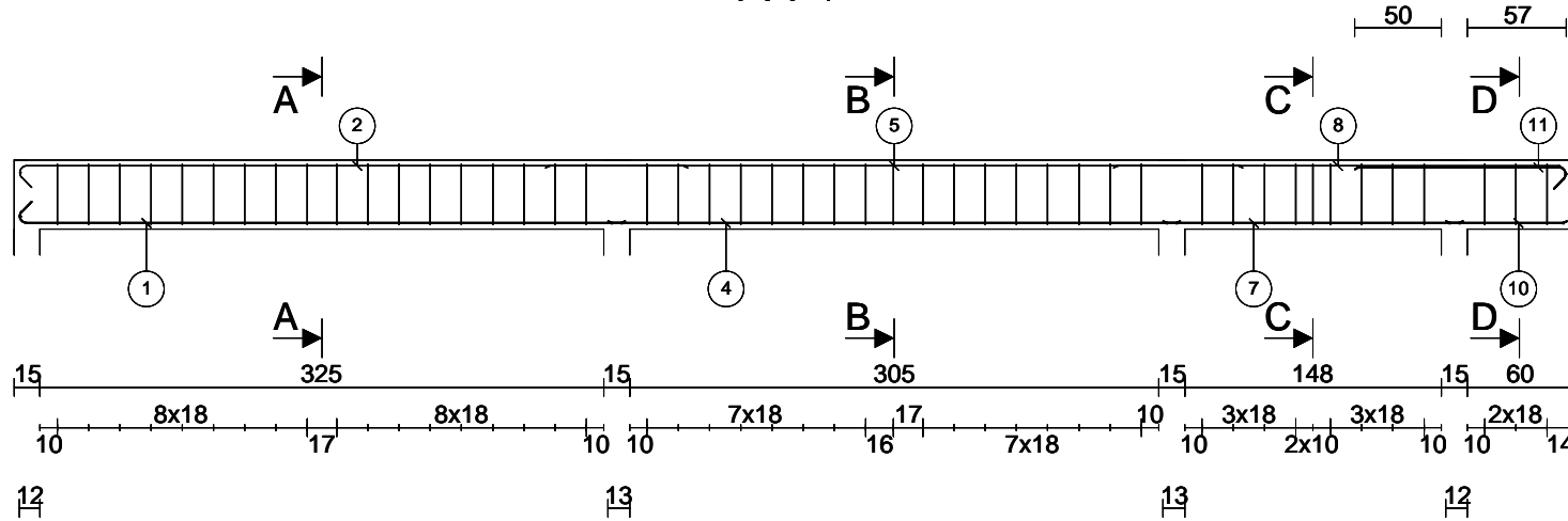
Élévation Echelle=1/47
