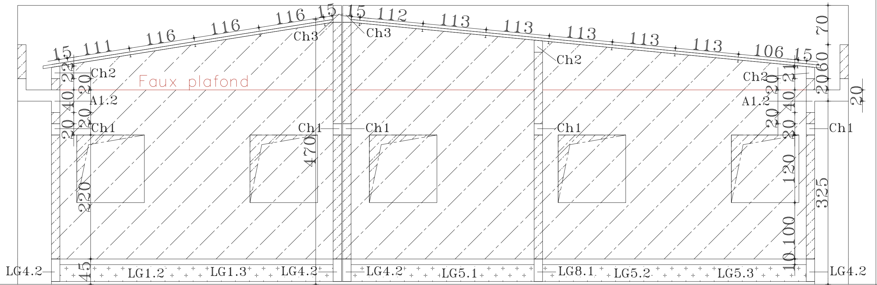
COUPE F-F
