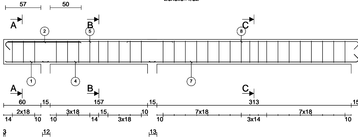
Elévation Echelle=1/32
