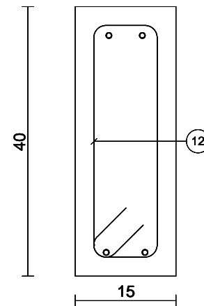
Coupe D-D Echelle=1/8
