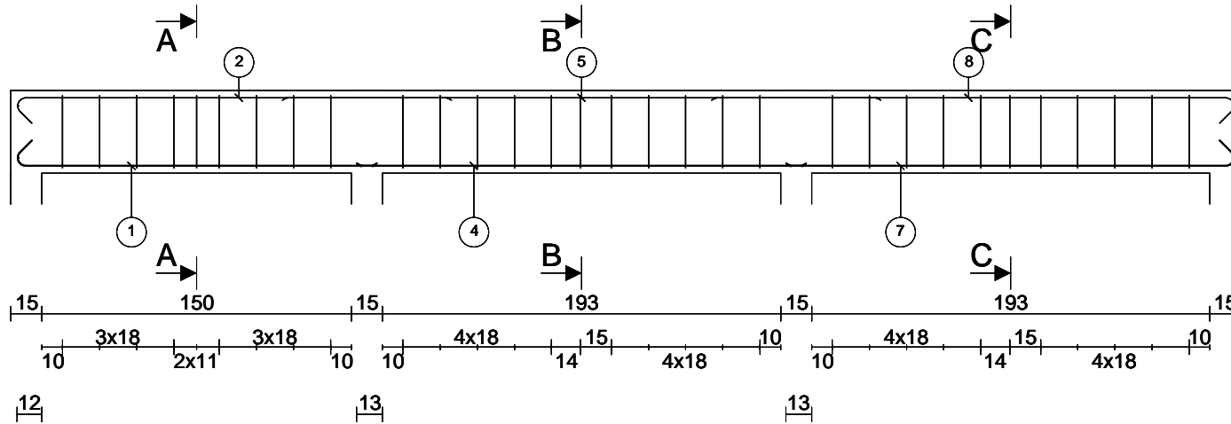
Elévation Echelle=1/33
