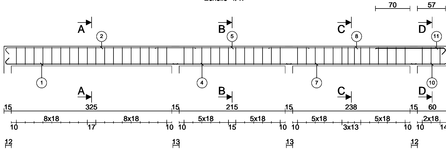
Elévation Echelle=1/47
