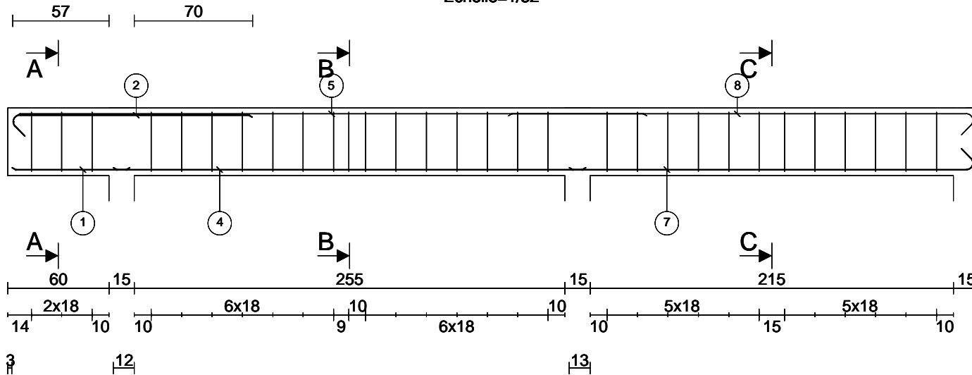
Elévation Echelle=1/32
