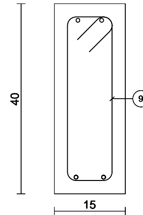
Coupe C-C Echelle=1/8
