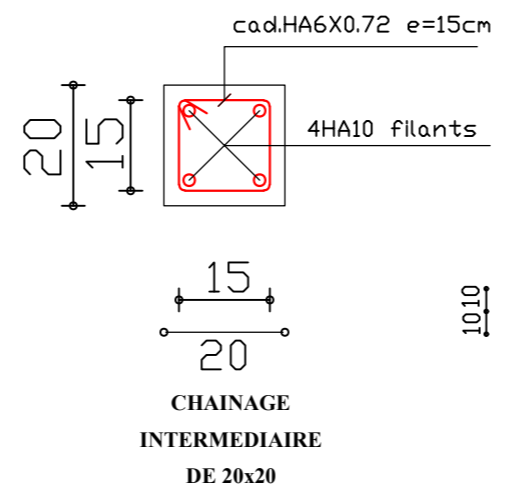
COUPE DETAIL 5-5 (Renfort de dallage)
