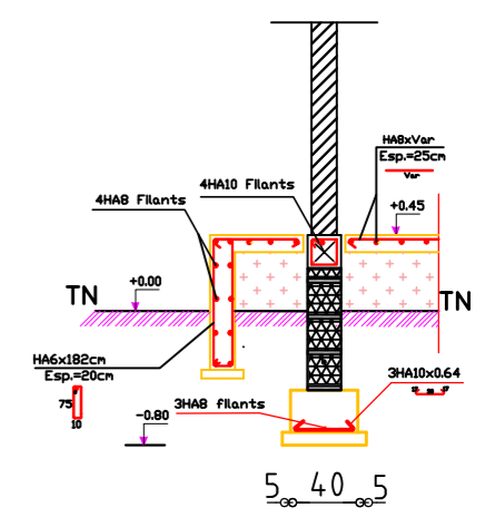
COUPE DETAIL 1-1 Coffrage
