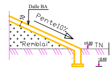
BECHE COUPE DETAIL 2-2 (Coffrage)
