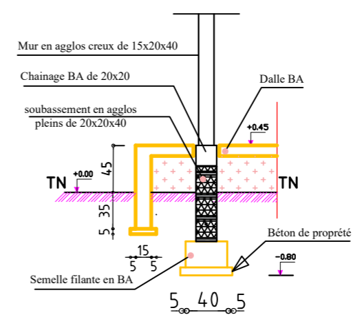
COUPE DETAIL 1-1 Coffrage
