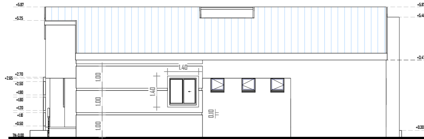
FACADE LATÉRALE DROITE
