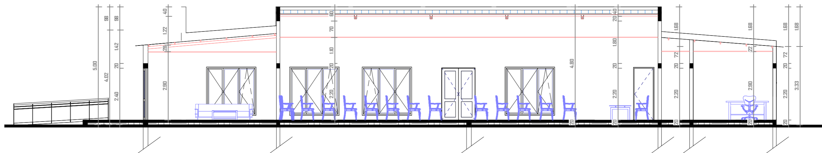
COUPE AA
