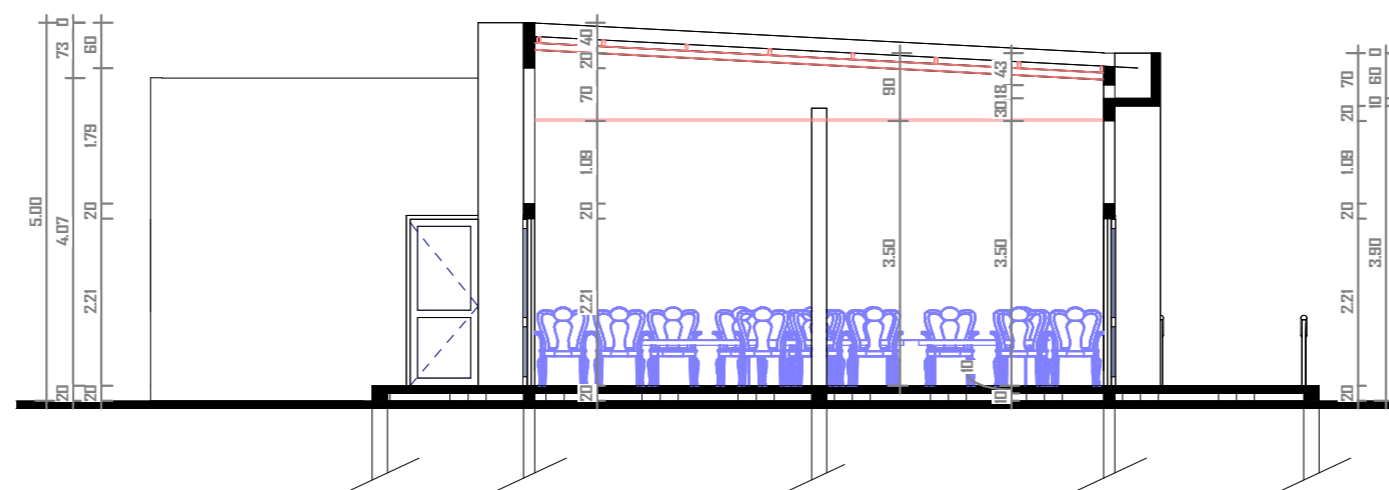
COUPE BB
