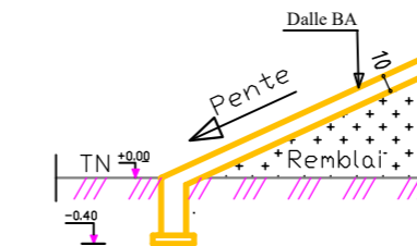
BECHE COUPE DETAIL 2-2 (Coffrage)
