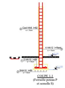
COUPE DETAIL 1-1
