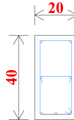
Coupe longrine
