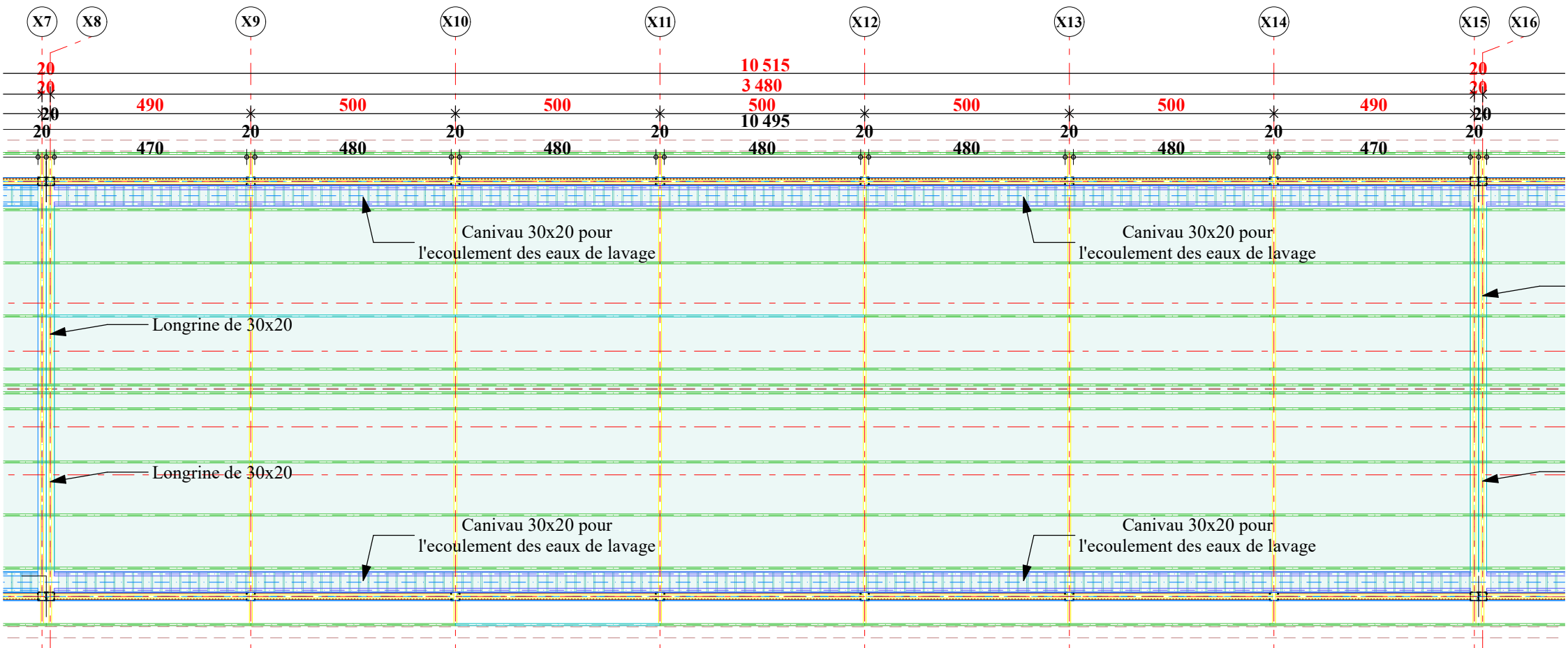
VUE EN PLAN
