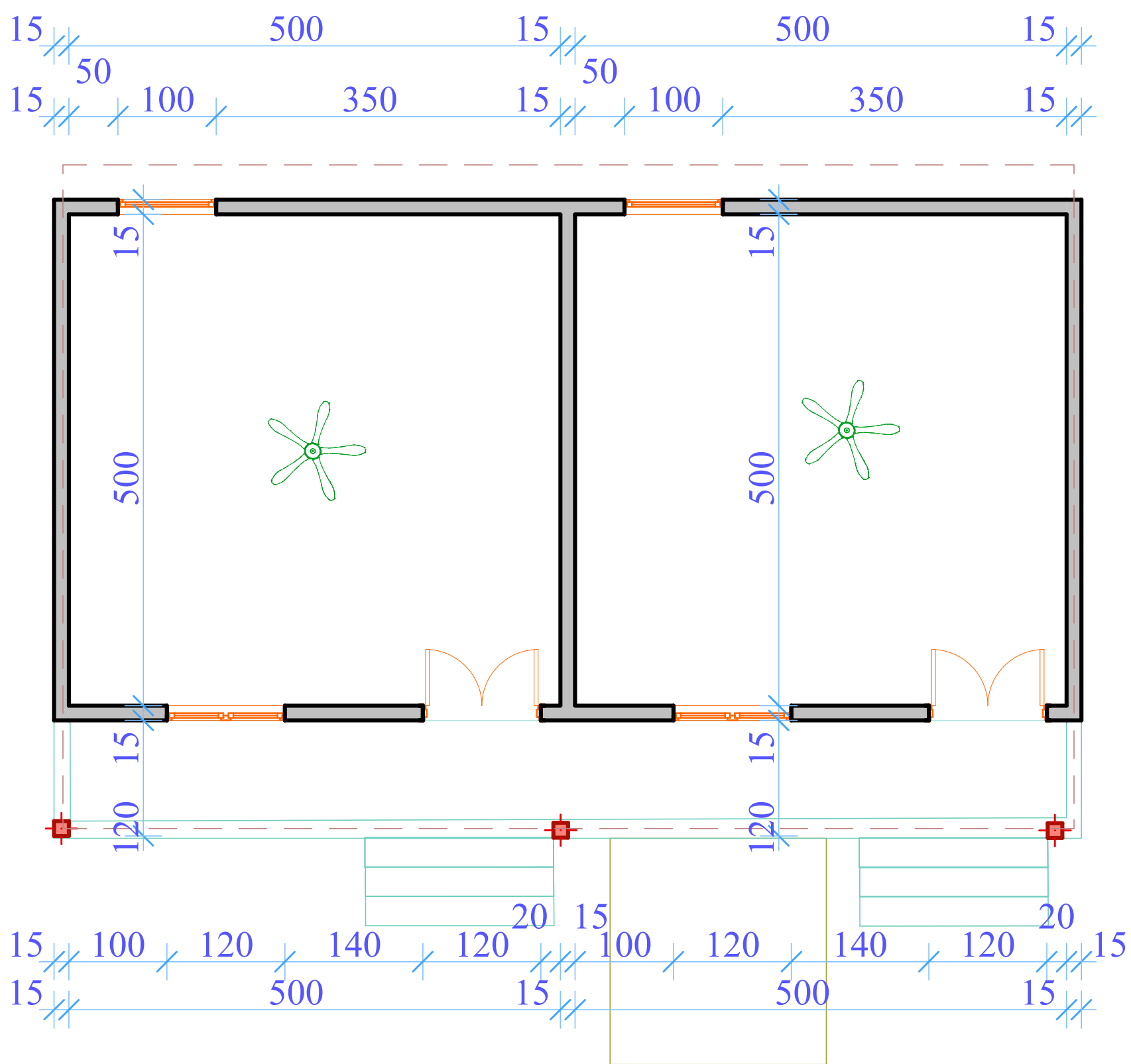
PLAN DE NIVEAU
