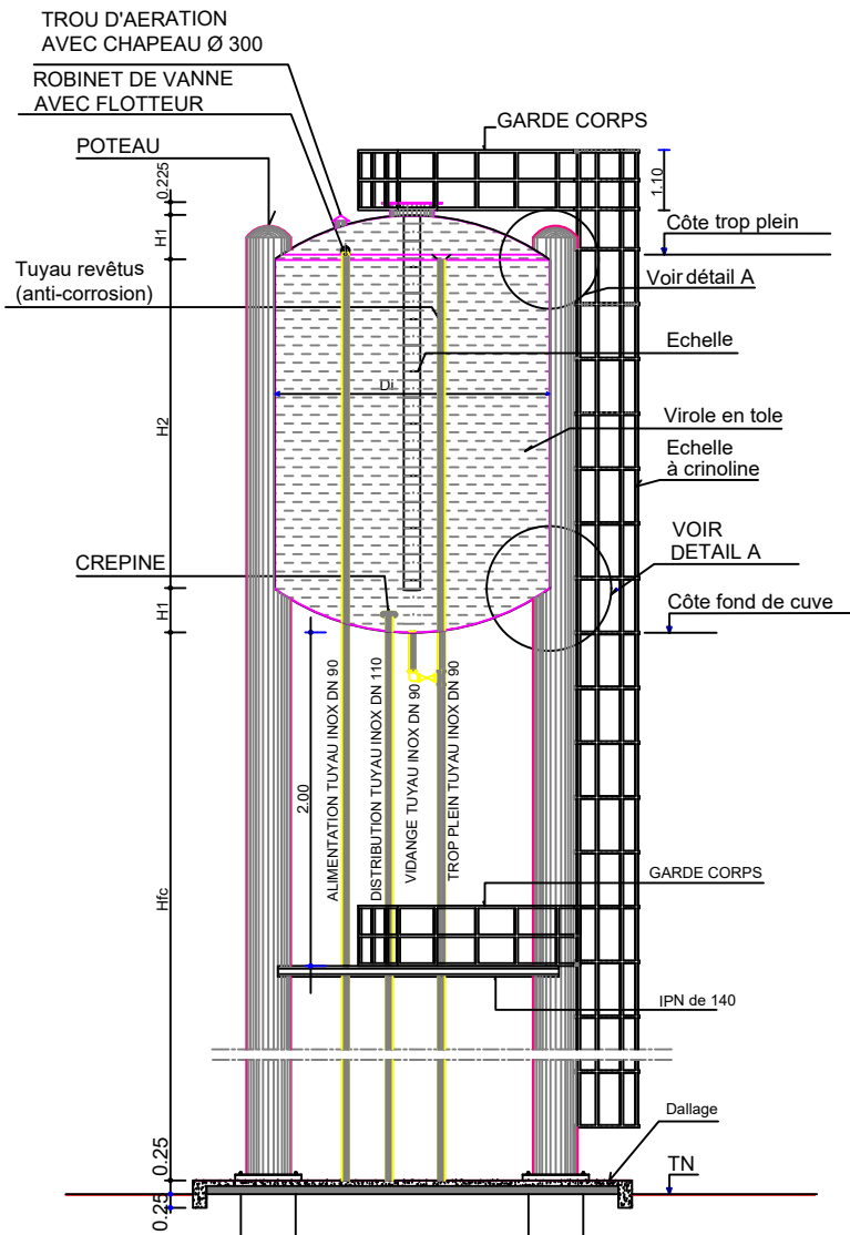
COUPE A - A
