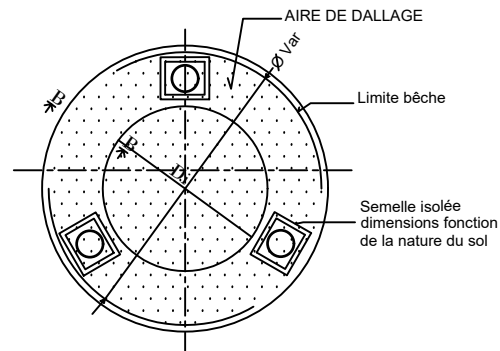
VUE EN PLAN-FONDATION
