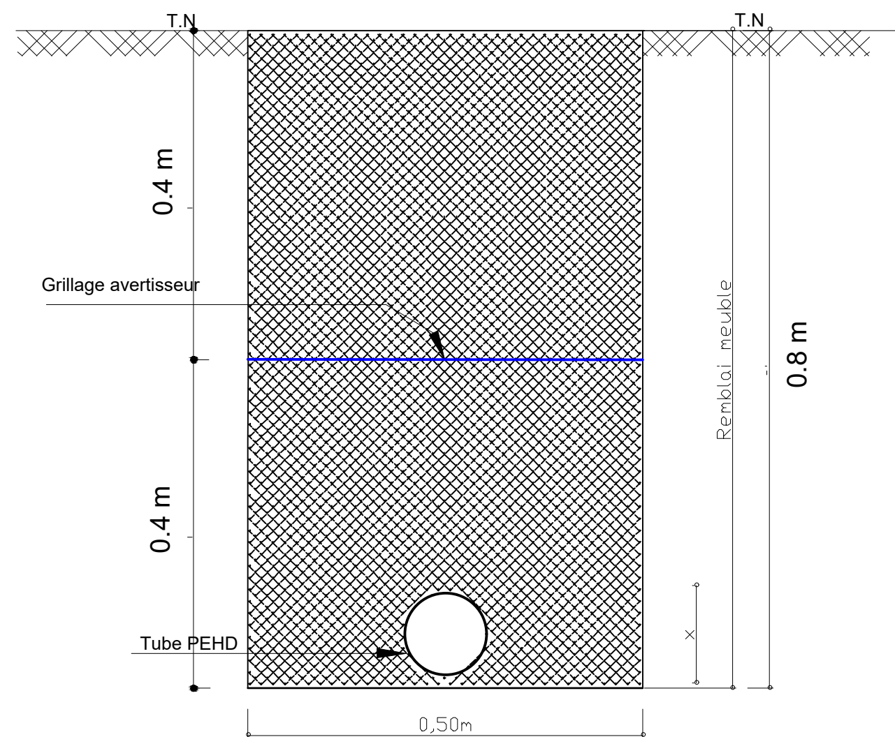
Pose en terrain normal
