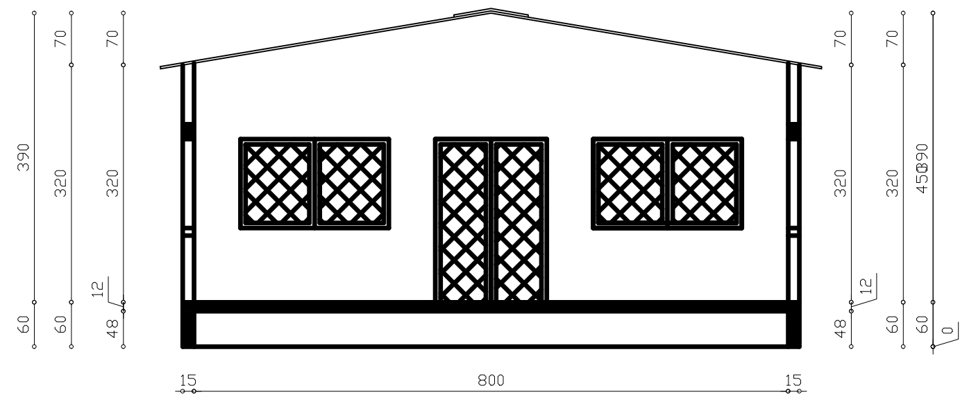
Coupe longitudinale
