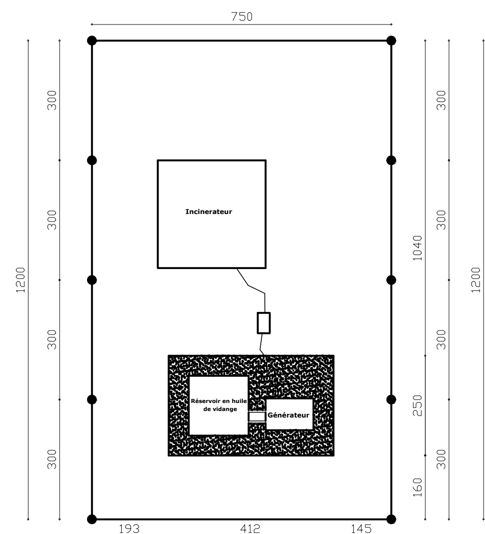
PLAN DE NIVEAU DU HANGAR
