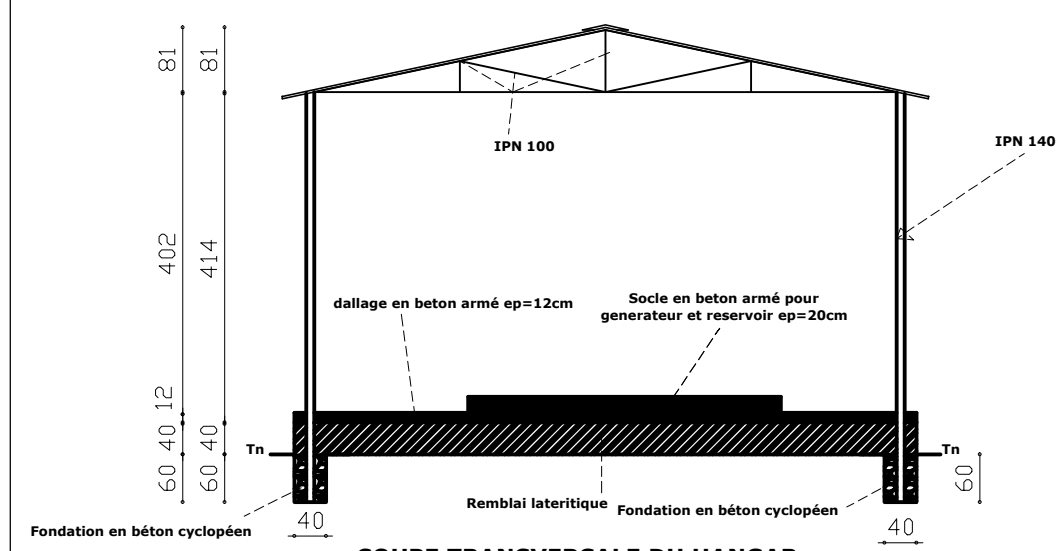
COUPE TRANSVERSALE DU HANGAR
