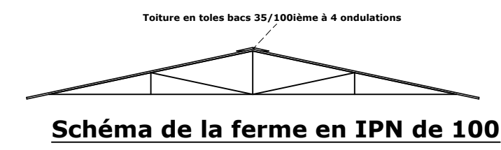
Fermes en deux versants( IPN de 100)
