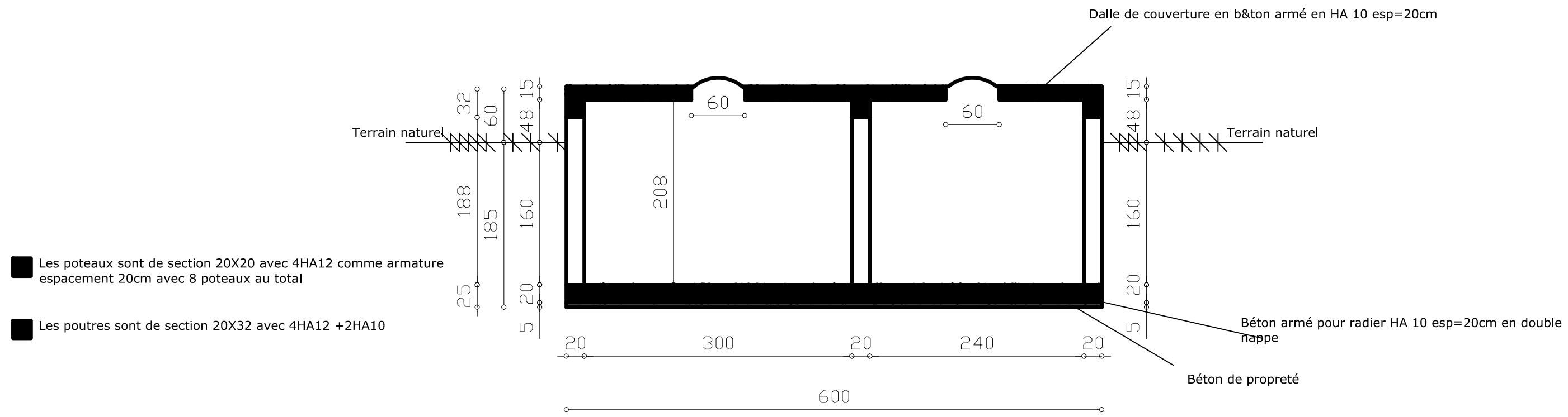
COUPE TRANSVERSALE DE LA FOSSE A CENDRE
